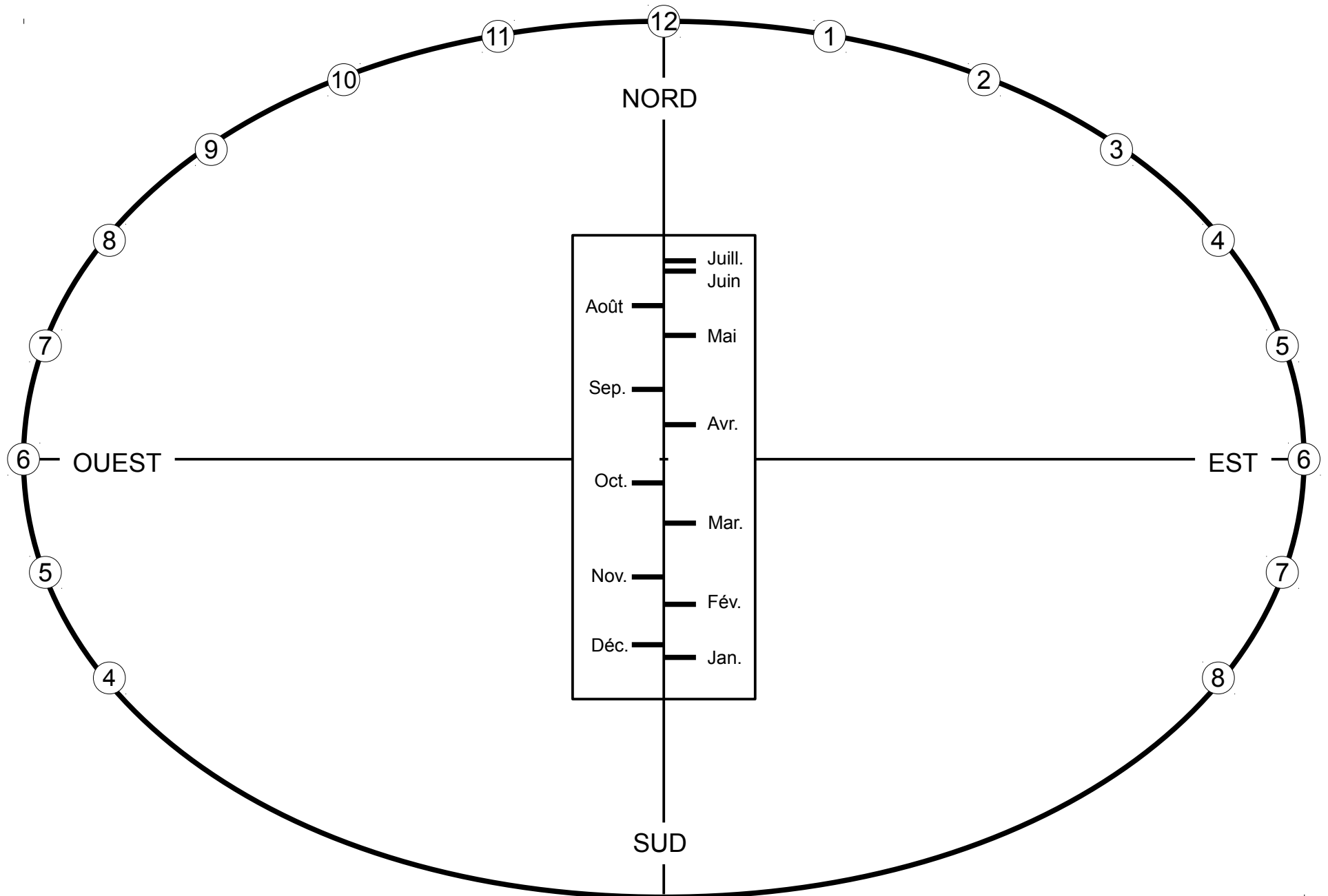
Cadran solaire analemmatique (Lat. 43° N)
